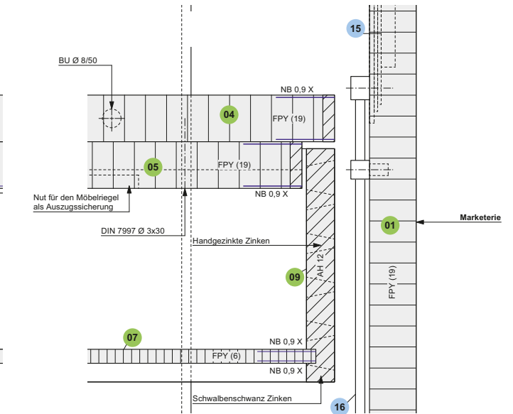
Die Marketerie mit den versetzten Spitzen der Rauten ist aufwendig zusammengesetzt
