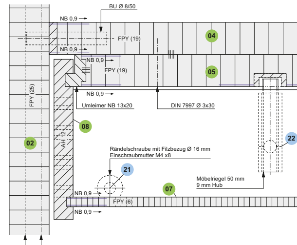
Frontalschnitt und Vertikalschnitt: Die beiden Schubkästen sind platzsparend ohne Mittelwand hängend geführt
